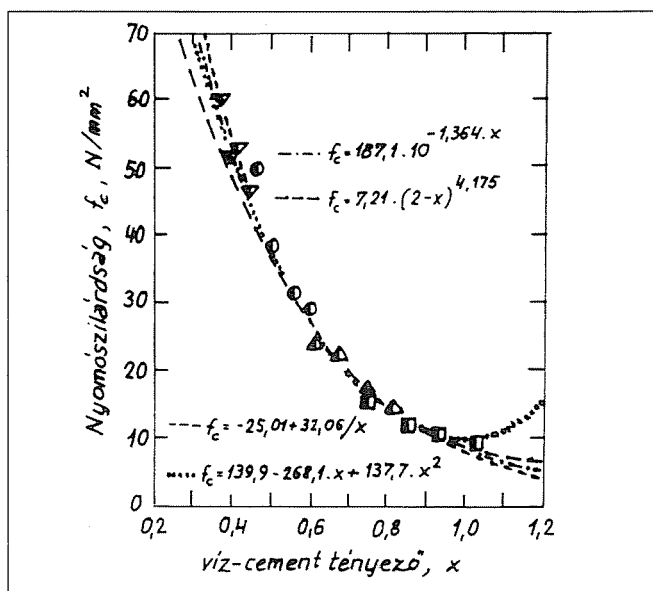
3. ábra: A víz-cement tényező alapuló, különböző alakú képletekkel becsült 28 napos nyomószilárdságok összehasonlítása (az adatok az 1. ábrából valók)
