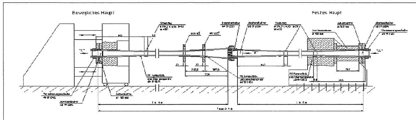
4. ábra: A statikus és a fáradási kísérlet általános elrendezése pászmás feszítőkábel esetén
